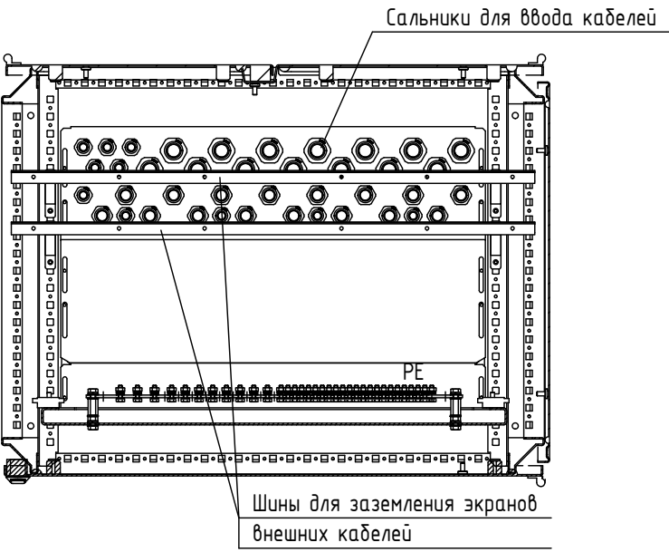
Б-Б
